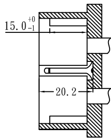
A--A(局部)
